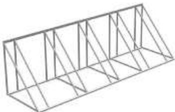
Велопарковка 5-ти местная "Гарби" Размеры: 2500х800х800 мм. Цена: 24 000 р.
