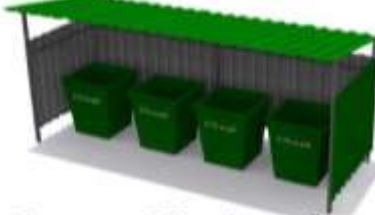
Площадка ТБО на 4 контейнера с навесом Размеры: 5200x1500x2000 мм. Цена: 93 000 р.
