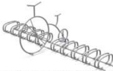
Велопарковка 10-ти местная "Энтон" Размеры: 4000х1200х1200 мм. Цена: 26 000 р.
