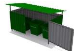
Площадка ТБО на 3 контейнера с навесом и воротами Размеры: 4000x1500x2000 мм. Цена: 95 000 р.
